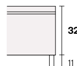
Giroletto/Bedframe H 32 cm Piede alto High feet
